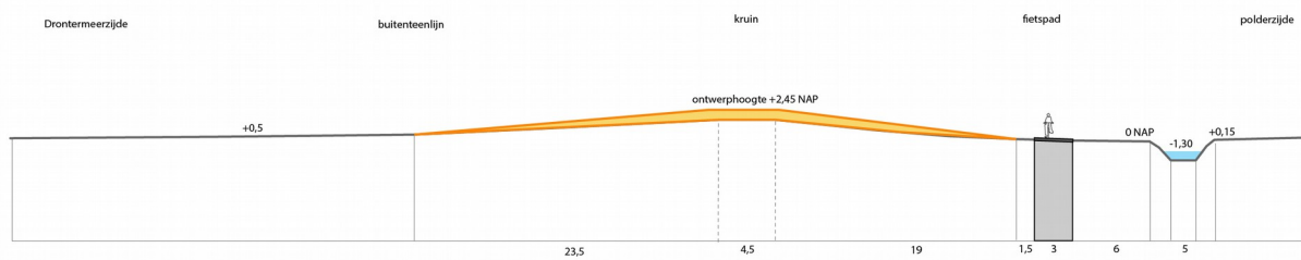
Figuur 3: Dwarsdoorsnede Voorkeursalternatief
